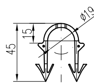
type D
