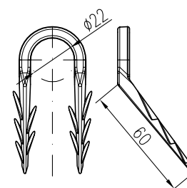
type E
